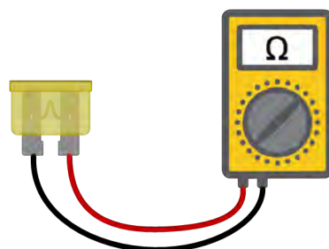
Durchgangsprüfung
